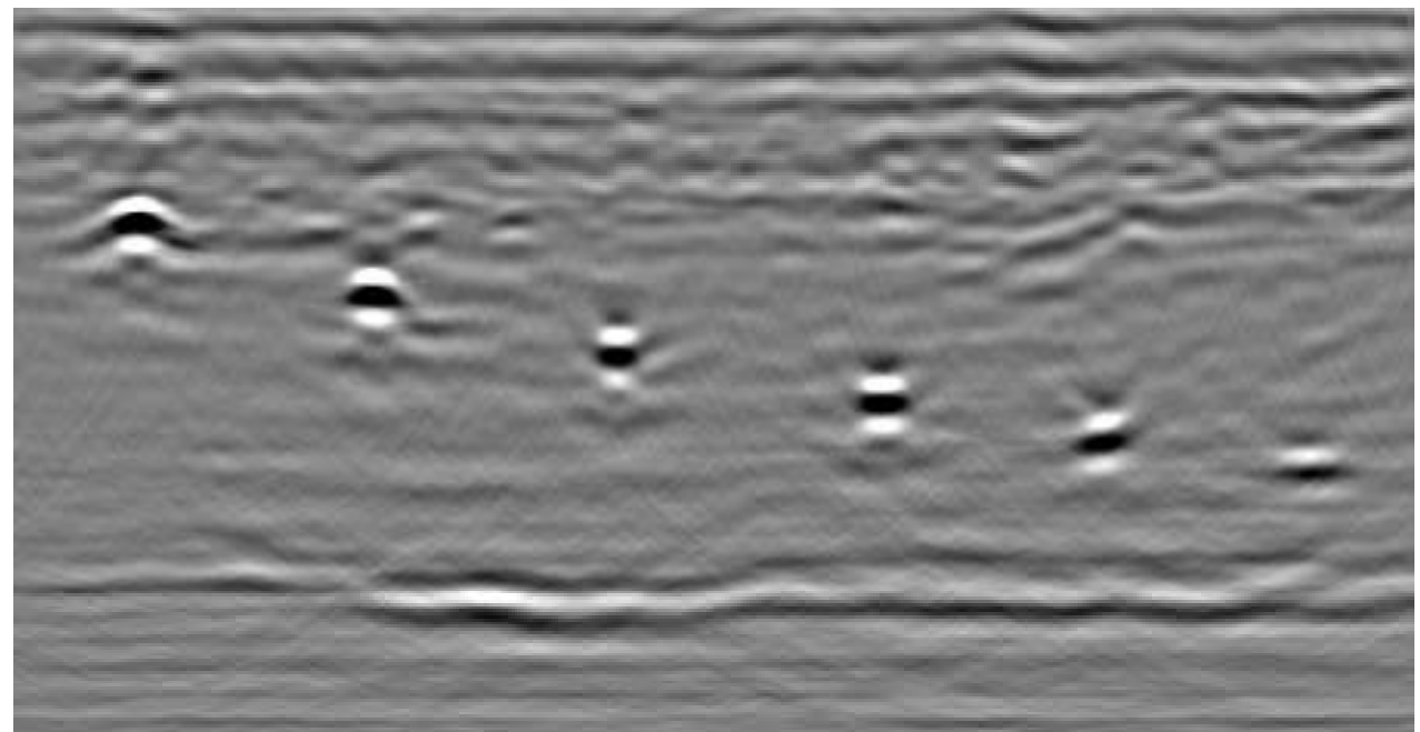
図2 f-kマイグレーション処理を行った波形
